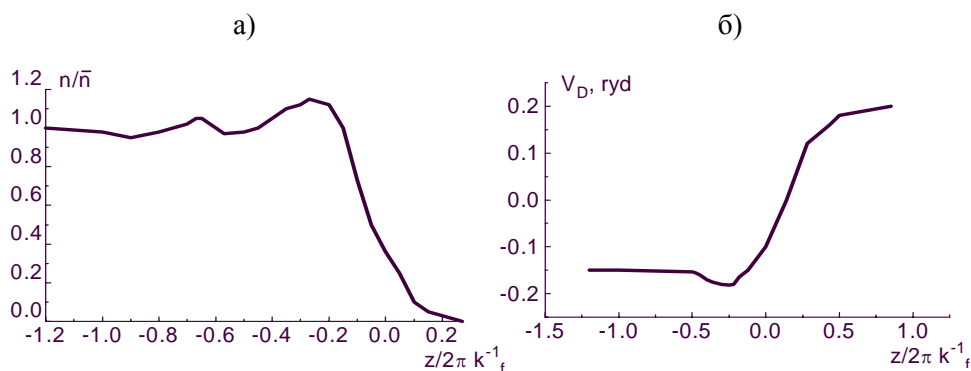
Рис. 1. Розподіл а) відношення концентрацій n/\bar{n} носіїв та б) потенціалу дипольного шару V_D у напрямку нормалі до поверхні (за даними [7,8])
